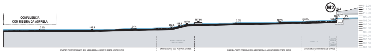
Perfil longitudinal da Ribeira da Manga com indicação dos açudes propostos
